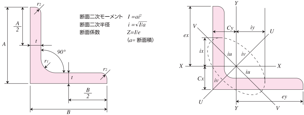
■断面寸法、断面積、単位質量及び断面特性
